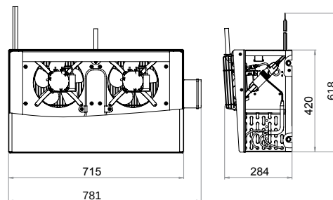
Внутренний блок
