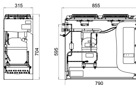
Внешний блок
