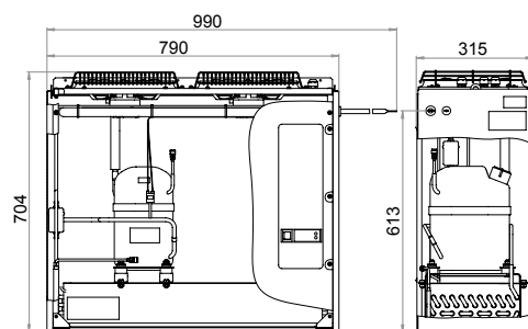
Внешний блок
