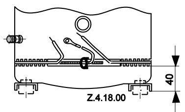
Рис 12: Размещение нагревателя картера
