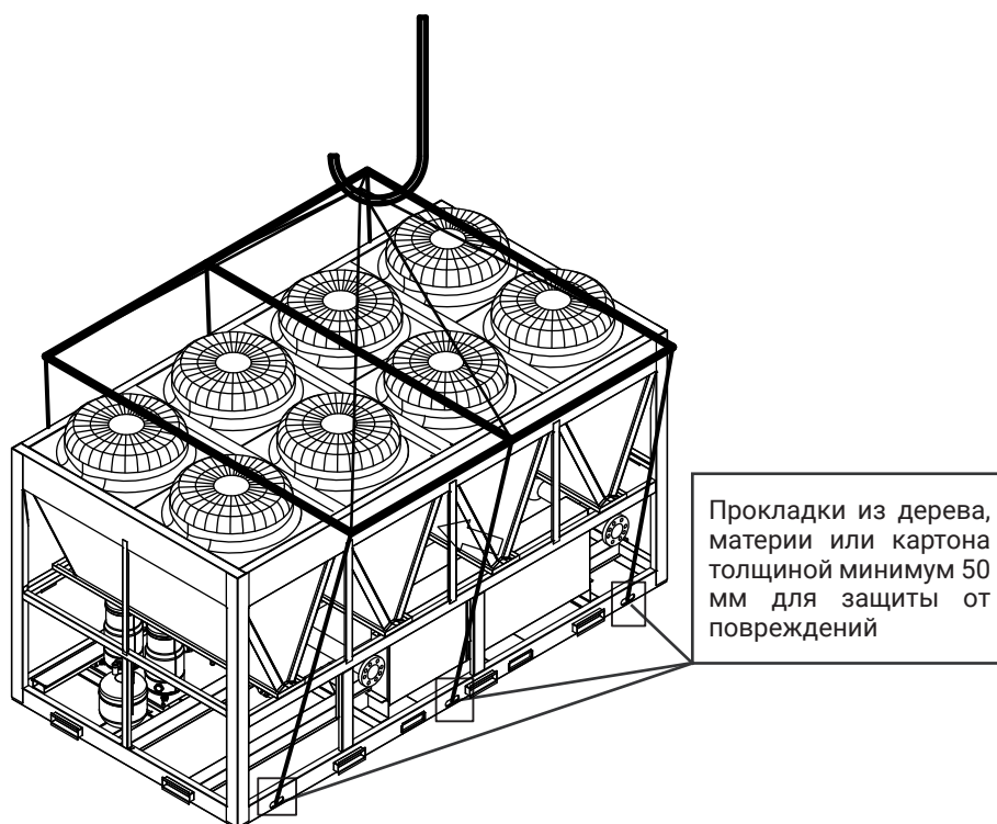
Рис. 4-1 Подъем установки
