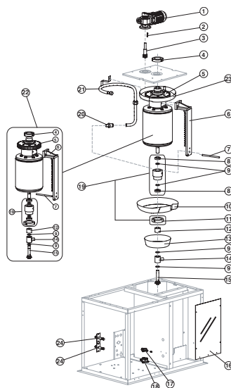
EVAPORATOR
