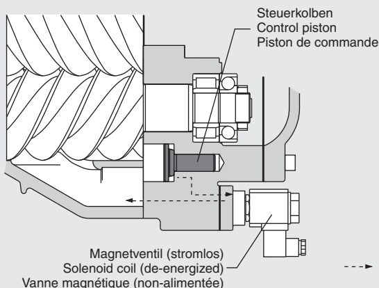
Konstruktiver Aufbau der Leistungsregelung (Anlaufentlastung)
