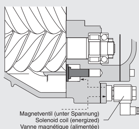
Détails de construction de la régulation de puissance (démarrage à vide)
