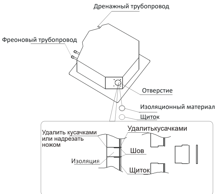
тип корпуса 1
